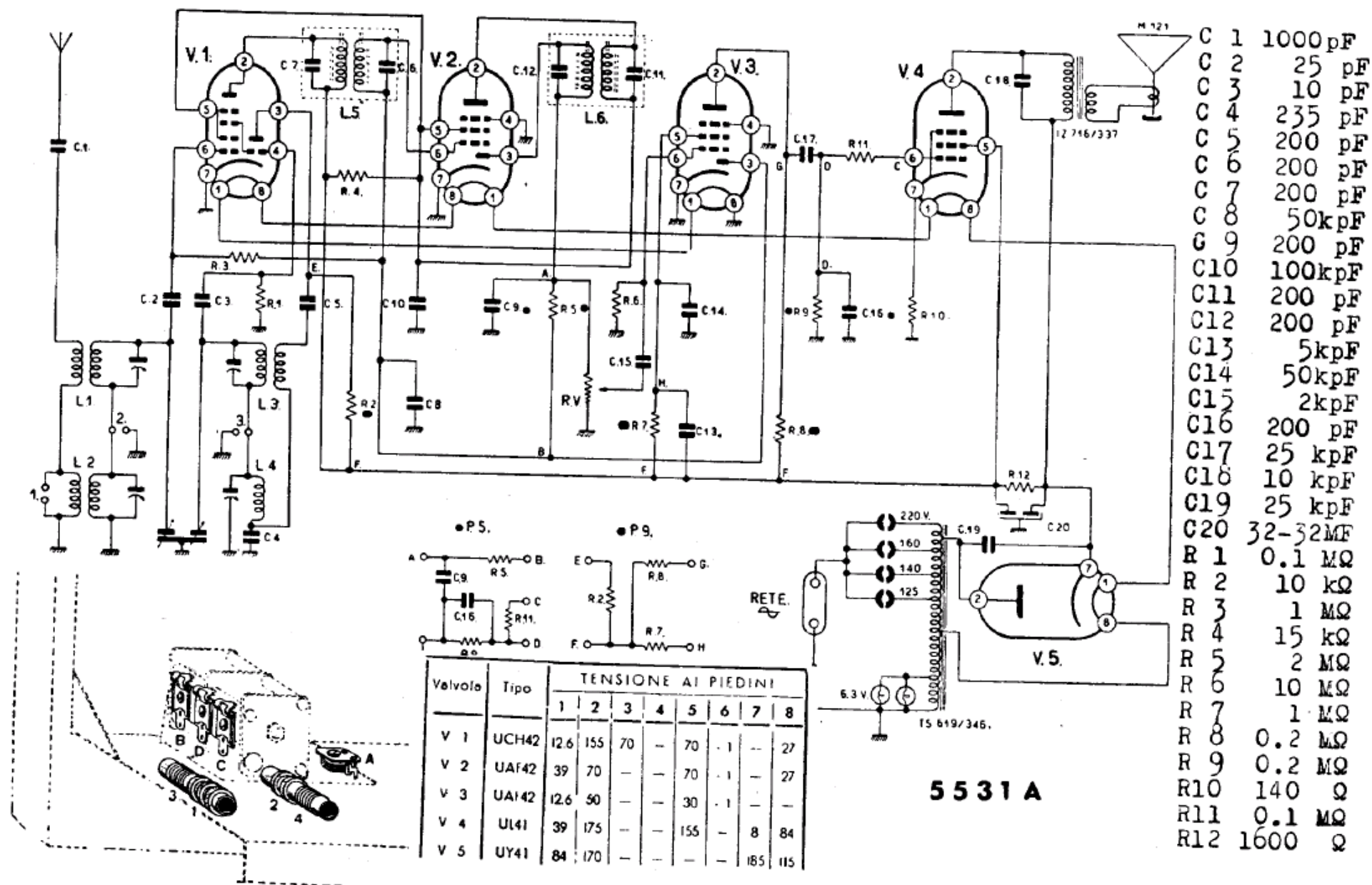
S.A. FIMI - Mod. PHONOLA 5531 A - Media frequenza 470 kc. Finale: 175 V placca, 155 V schermo e 8 V catodo. Potenza indistorta 2 watt. Consumo 35 watt. (V. istruzioni funicella a parte).
